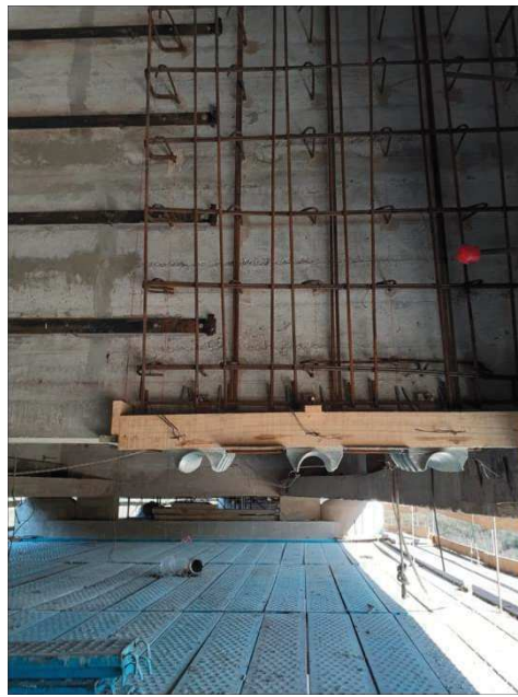
2-10 Armado de refuerzos transversales, colocación de piezas desviadoras
