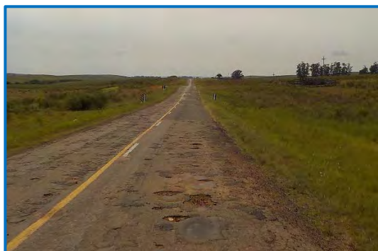
Situación típica de la calzada previo a la rehabilitación.
