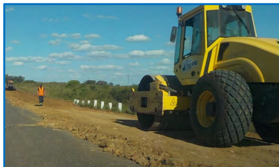
Recargo y compactación de material granular.
