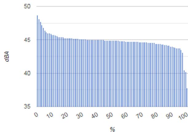
Curvas de permanencia para cada punto medido
