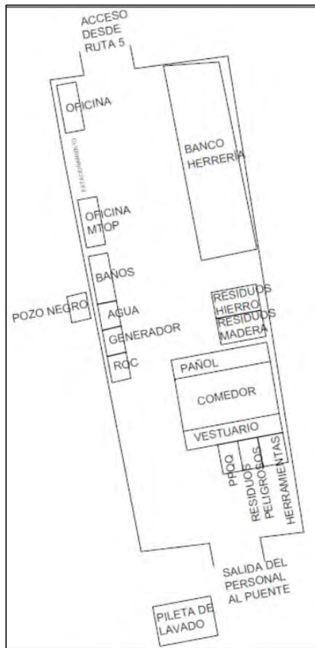
Figura 2-3 Ubicación y esquema obrador pasaje ferroviarios en km 120 (La Cruz)
