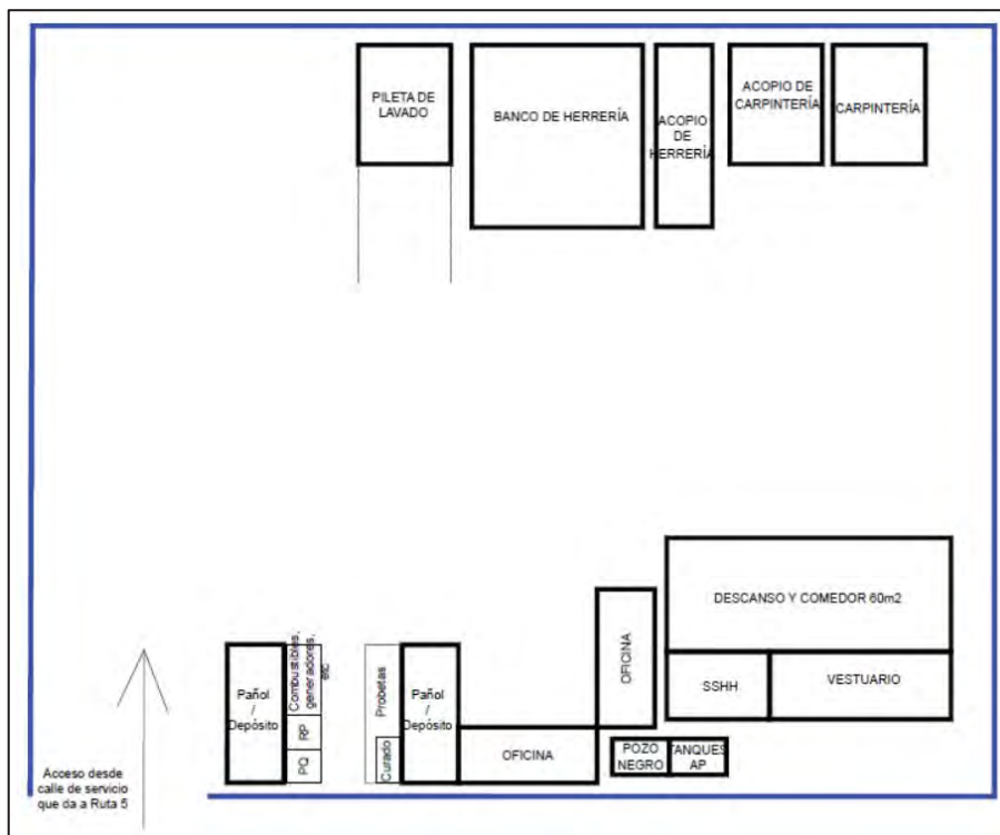
Figura 2-2 Ubicación y esquema obrador viaducto camino 60
