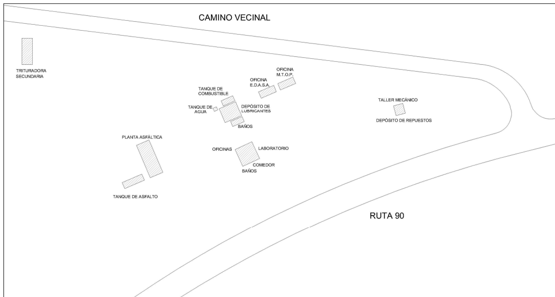
Plano de distribución del obrador
