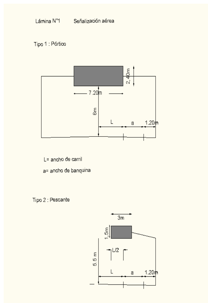
Imagen 2. Dimensiones a considerar para la señalización aérea.
